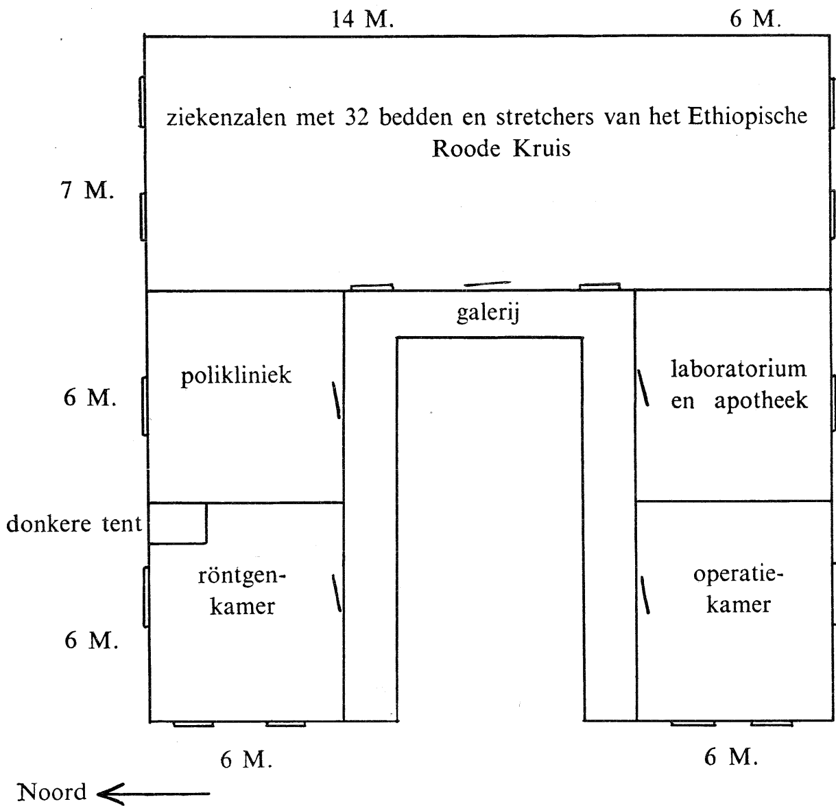
Fig. 9. Plattegrond van het basishospitaal der Ambulance in Ethiopië van het Nederlandsche Roode Kruis, in een der gebouwen van de Fransche Missie te Dessié.
